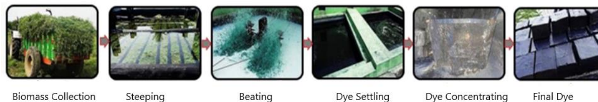
شکل ۶: فرآیند استخراج ایندیگو [۵۹]
