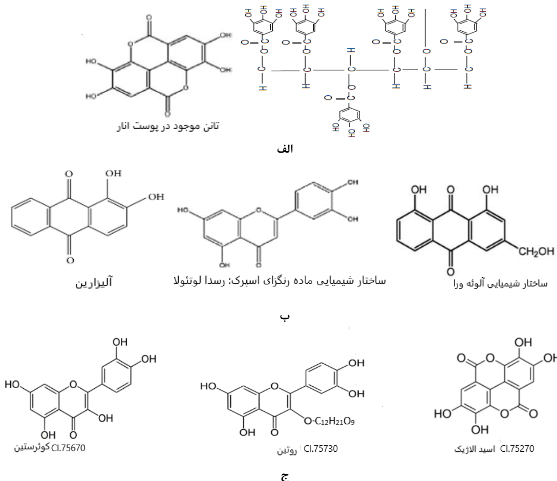
شکل ۵: ساختار شیمیایی الف: تانن‌های محلول در آب، ب: آلوه ورا، روناس و اسپرک و ج: ساختارهای شیمیایی موجود در گیاه اکالیپتوس [۹۰، ۱۷، ۲۱، ۲۵].
